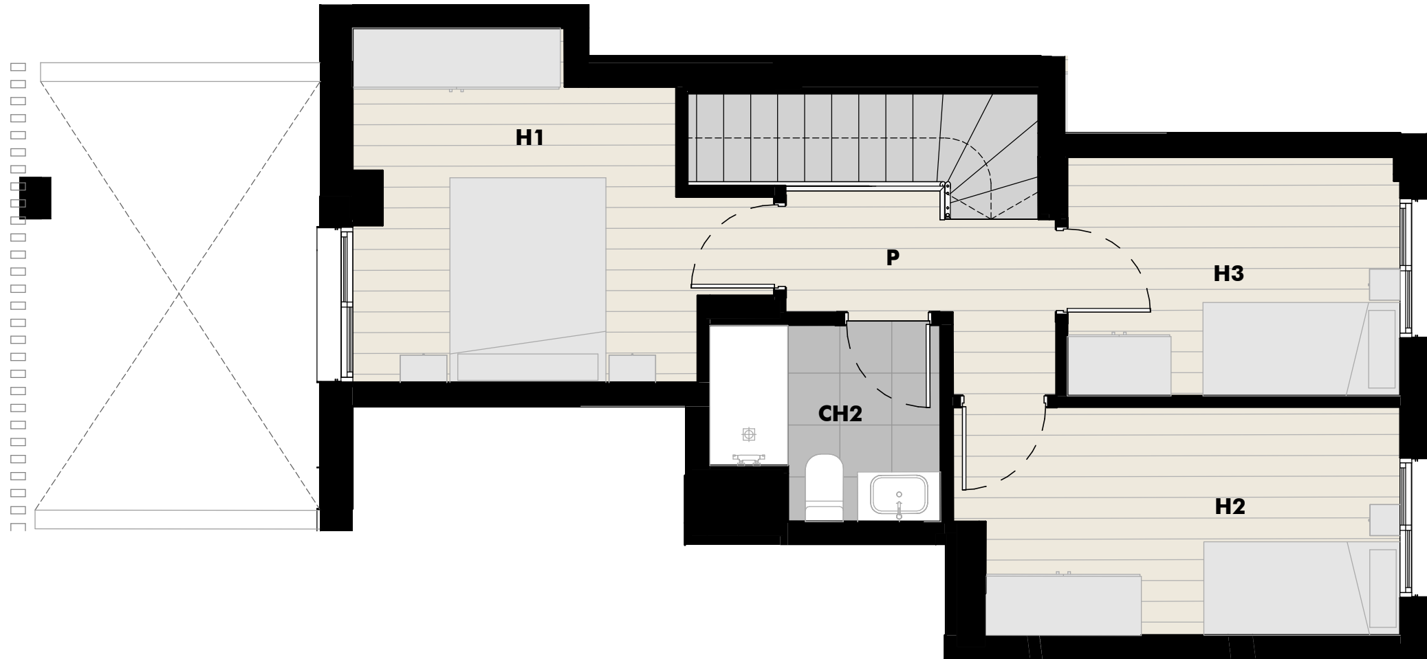
PLANTA ALTELL
